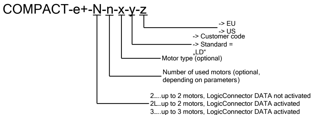
Abbildung 8: Bestellcode
