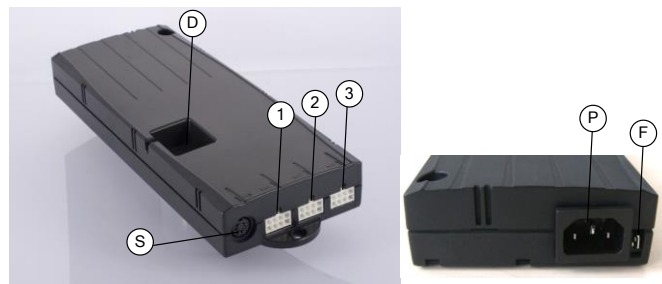
Abbildung 2: Buchsen
