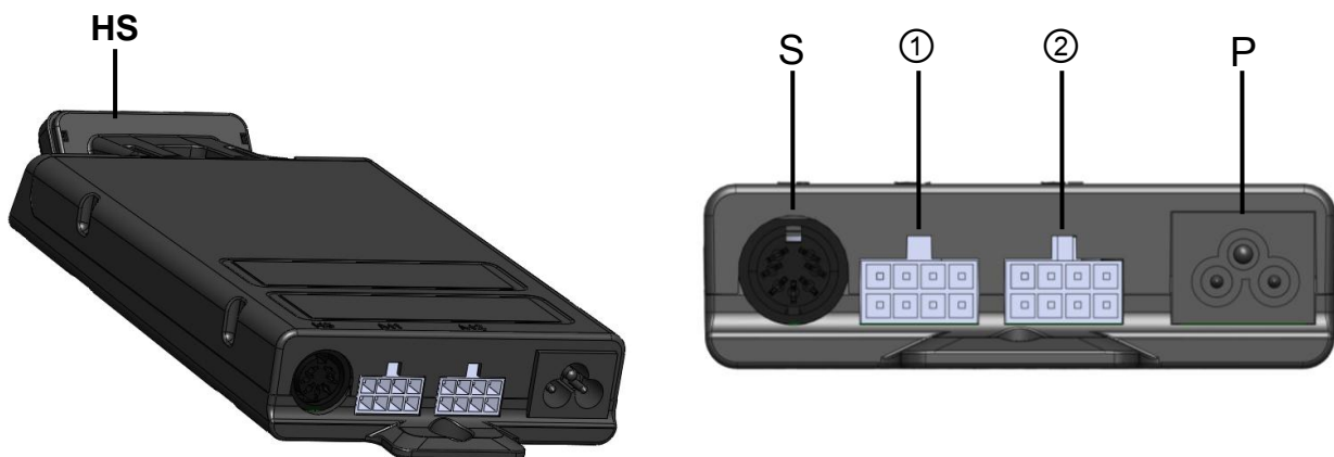
Abbildung 2: Buchsen
