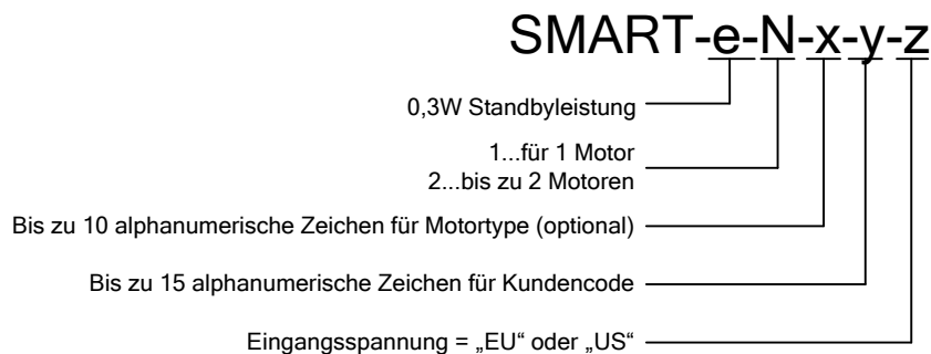
Abbildung 10: Bestellcode
